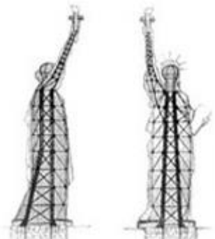
Armature de la statue de la Liberté
